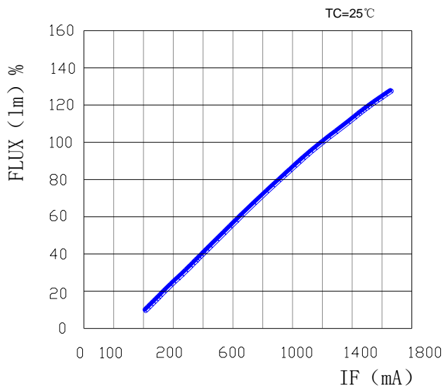
正向电流 VS. 亮度关系图
